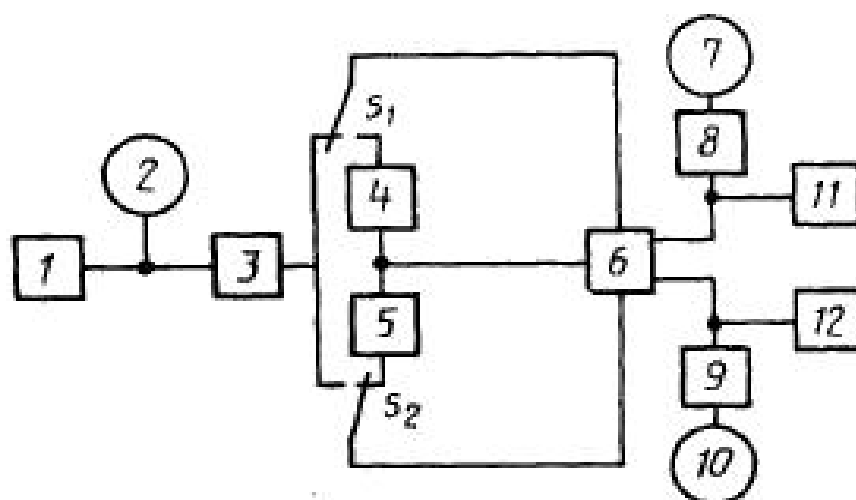
1 — генератор; 2, 7, 10 — вольтметры; 3 — согласующее звено; 4, 5 — эквиваленты сопротивления источника; 6 — измерительный усилитель; 8, 9 — фильтры; 11, 12 — эквиваленты нагрузки; S_1, S_2 — переключатели
