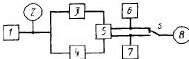
1 — генератор; 2, 8 — вольтметры; 3, 4 — эквиваленты полного сопротивления источника; 5 — измеряемый усилитель; 6, 7 — эквиваленты нагрузки; 5 — переключатель
